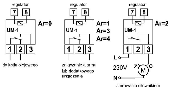
Rysunek 3. Schematy podłączenia modułu UM-1.
