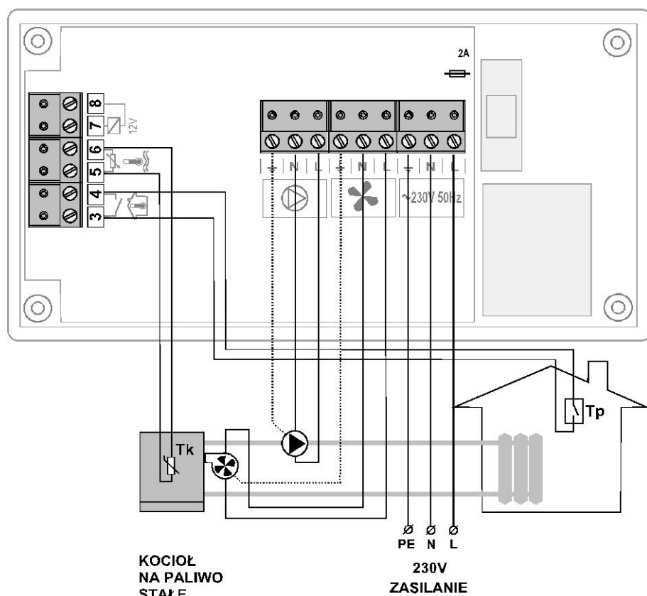
Rysunek 2. Schemat podłączenia regulatora RK-2001T2.
