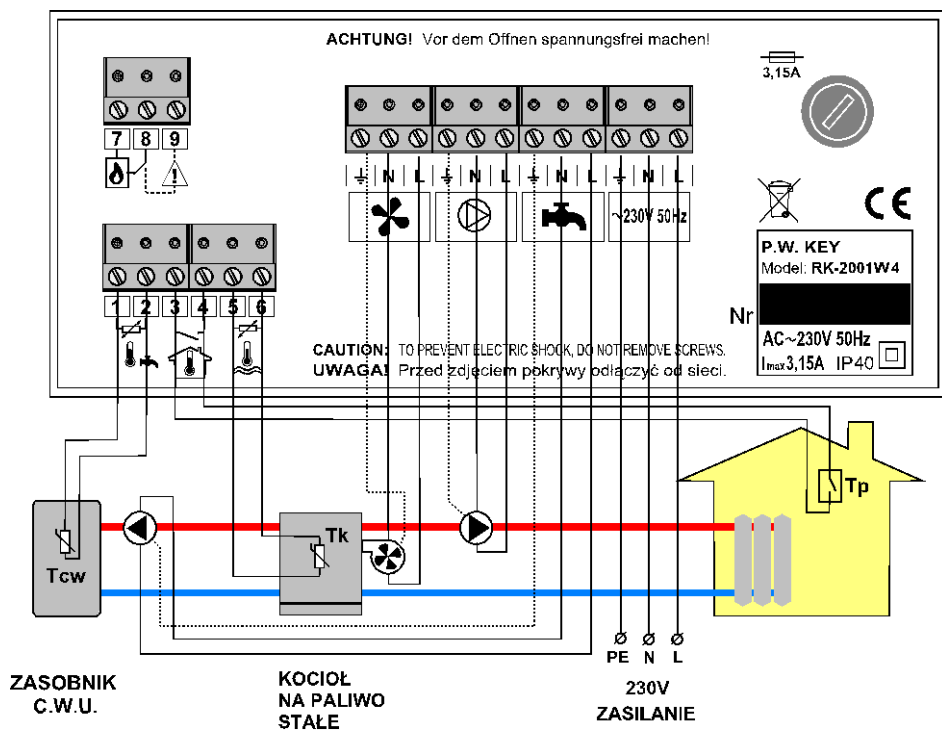
Rysunek 2. Schemat podłączenia regulatora RK-2001W4.
