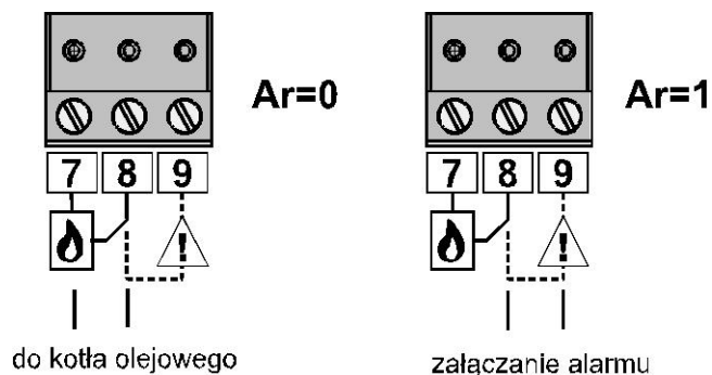
Rysunek 3. Schematy podłączenia urządzeń dodatkowych.
