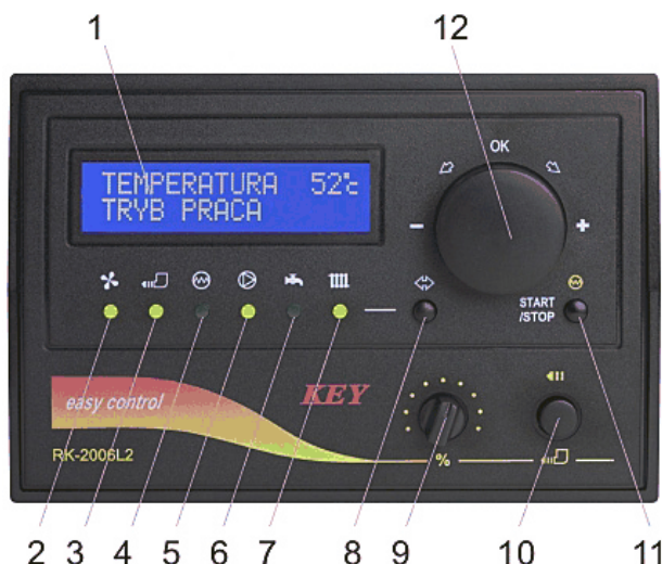
Рис. 1. Передняя панель контроллера RK-2006L2
