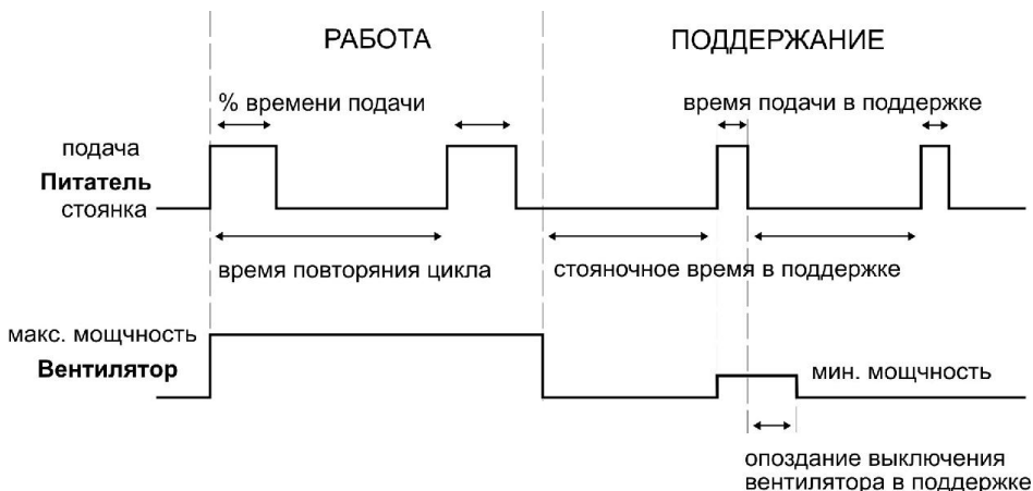
Рисунок 2. Принцип действия питателя и вентилятора.
