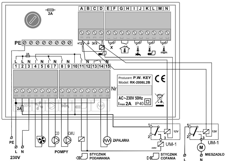
Rysunek 3. Schemat podłączenia regulatora RK-2006L2B.
