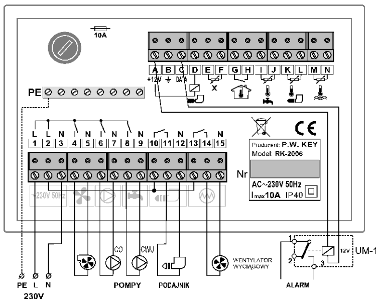
Rysunek 3. Schemat podłączenia regulatora RK-2006L2U
