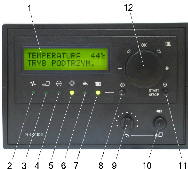
Rysunek 1. Płyta czołowa regulatora RK-2006L2U
