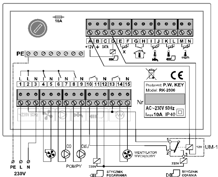
Rysunek 4. Schemat podłączenia regulatora RK-2006L2U z układem cofania paliwa
