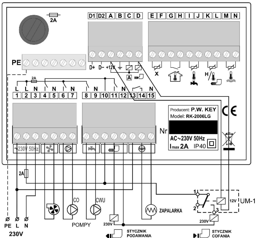
Rysunek 4. Schemat podłączenia regulatora RK-2006LG (z układem cofania paliwa).
