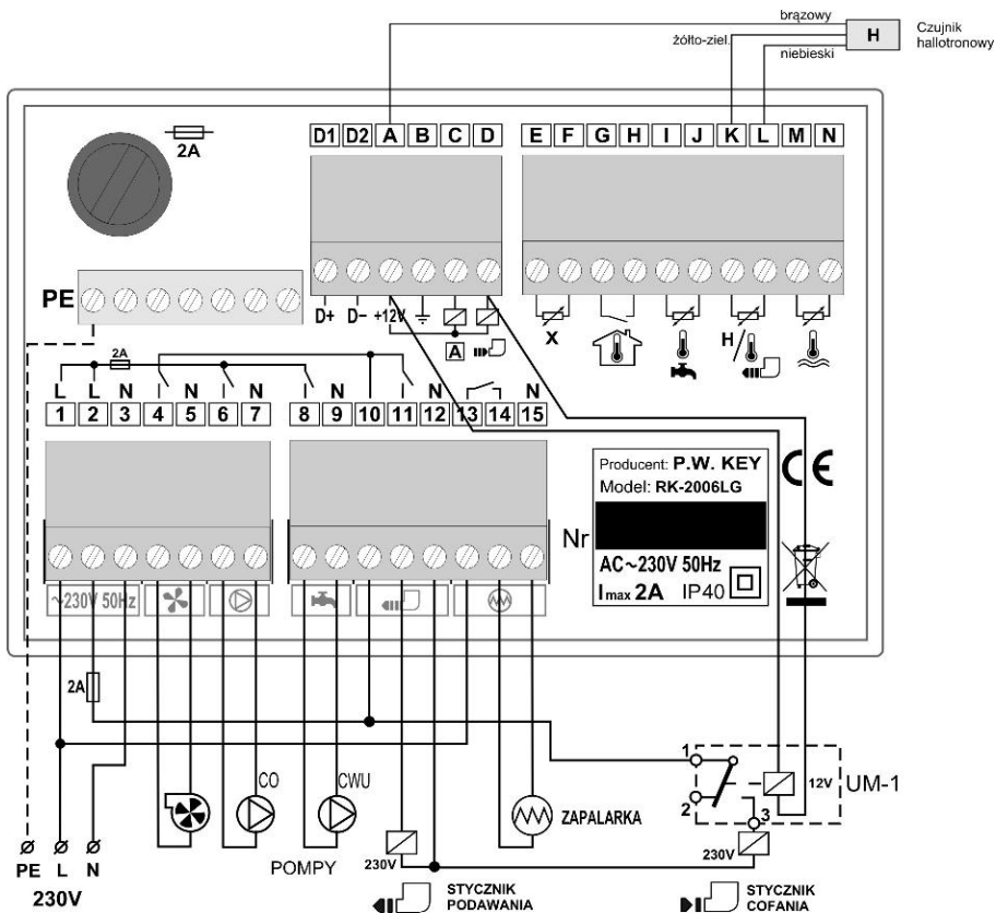
Rysunek 6. Schemat podłączenia regulatora RK-2006LG do kotłów z podajnikiem tłokowym (z układem cofania paliwa).
