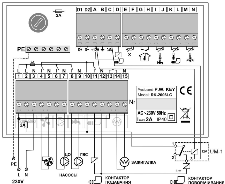
Рисунок 3. Схема подключения регулятора RK-2006LG (с системой поворачивания назад горючего).
