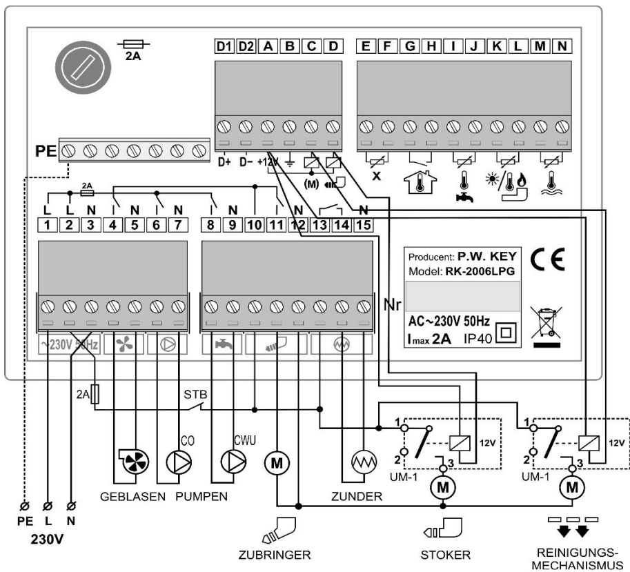
Abbildung 2. Anschlussschema des Reglers RK-2006LPG.
