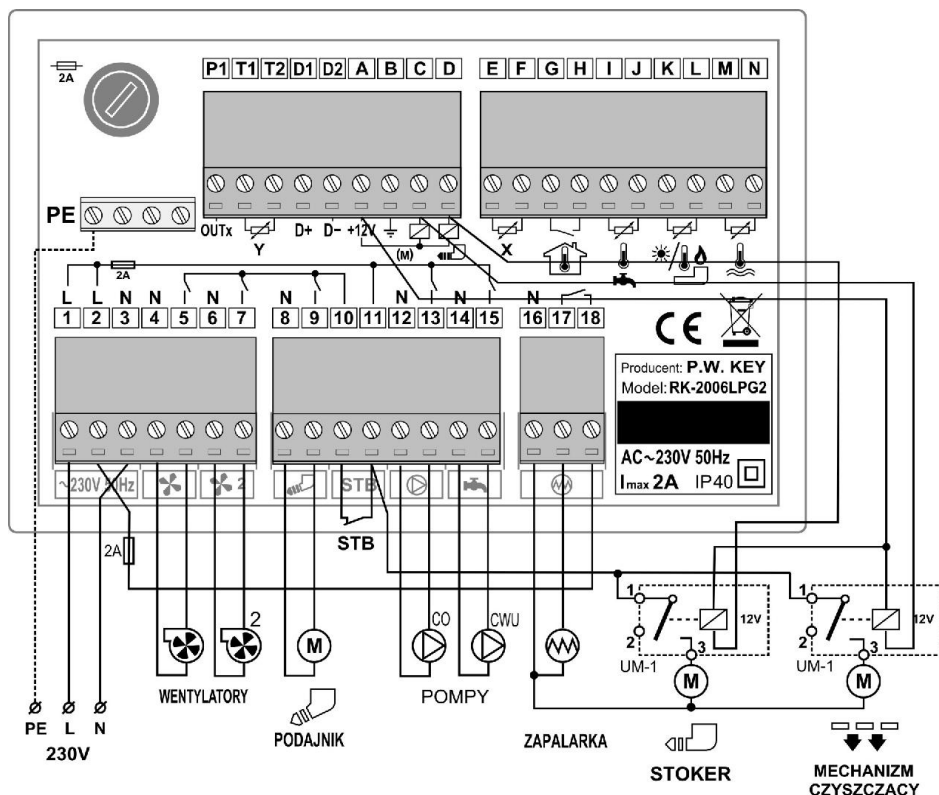
Schemat podłączenia regulatora RK-2006LPG2
