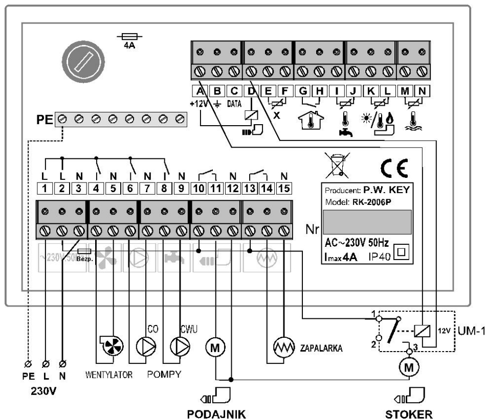
Rysunek 2. Schemat podłączenia regulatora RK-2006LPP.
