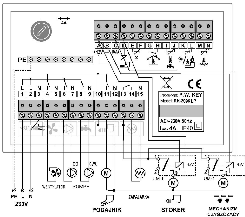
Rysunek 2. Schemat podłączenia regulatora RK-2006LPP.
