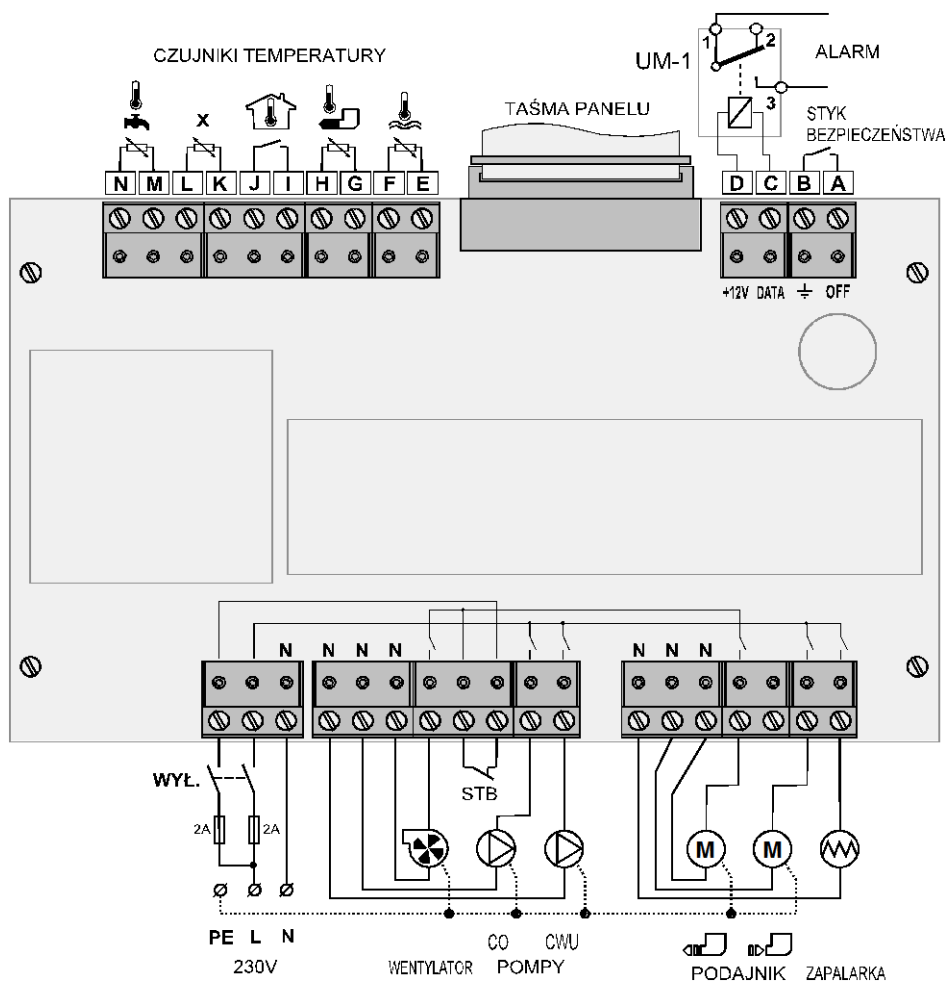
Rysunek 3. Schemat podłączenia zasilacza regulatora RK-2006LSC.
