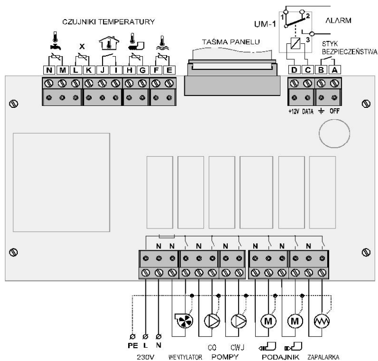
Rysunek 3. Schemat podłączenia zasilacza regulatora RK-2006LSz.
