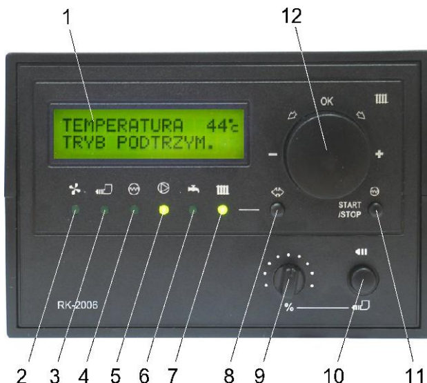
Rysunek 1. Płyta czołowa regulatora RK-2006LSZ
