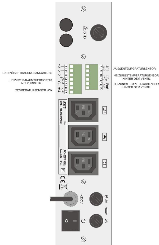
Anschlussplan des Reglers RK-2006SPGM mit Netzgerät MZL Version V.06.2015
