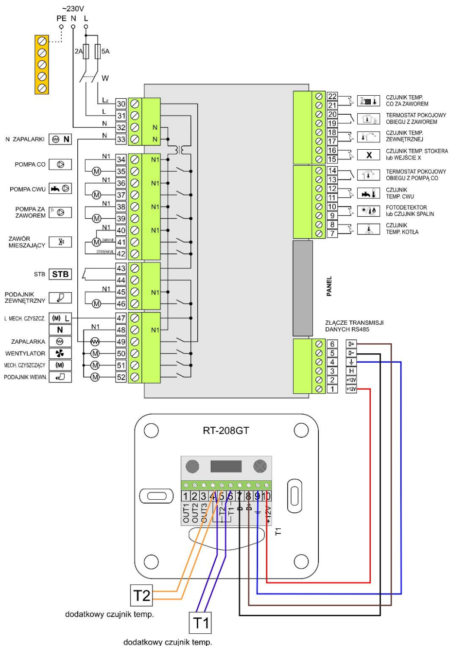
Schemat podłączenia regulatora RT-208GT do regulatora RK-2006SPGM z modułem zasilacza MZK, MZM2 wersja V.05.2018
