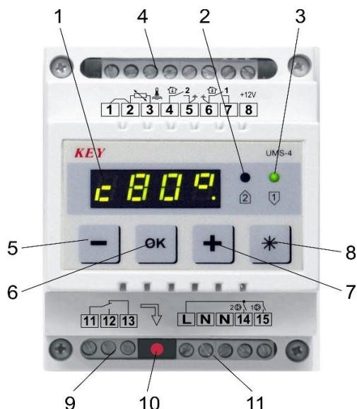
Rysunek 1. Widok płyty czołowej modułu UMS-4S2.
