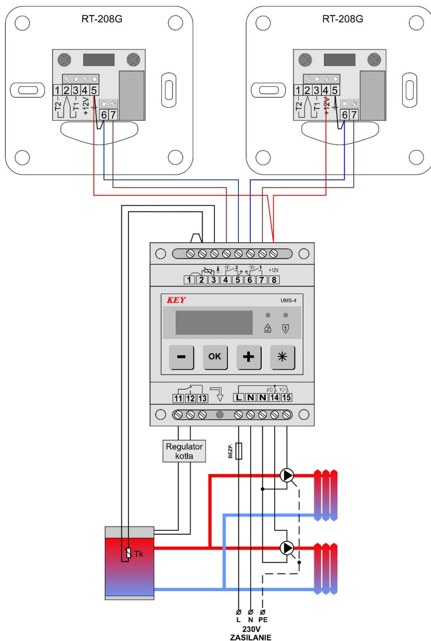
Rysunek 3. Schemat podłączenia modułu UMS-4S2 i termostatu pokojowego RT-208G.
