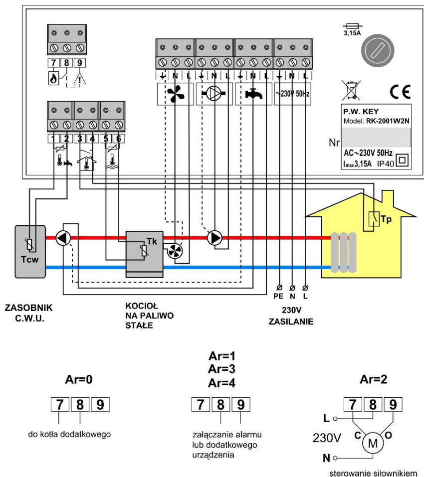
Rysunek 2. Schemat podłączenia regulatora RK-2001W2N.
