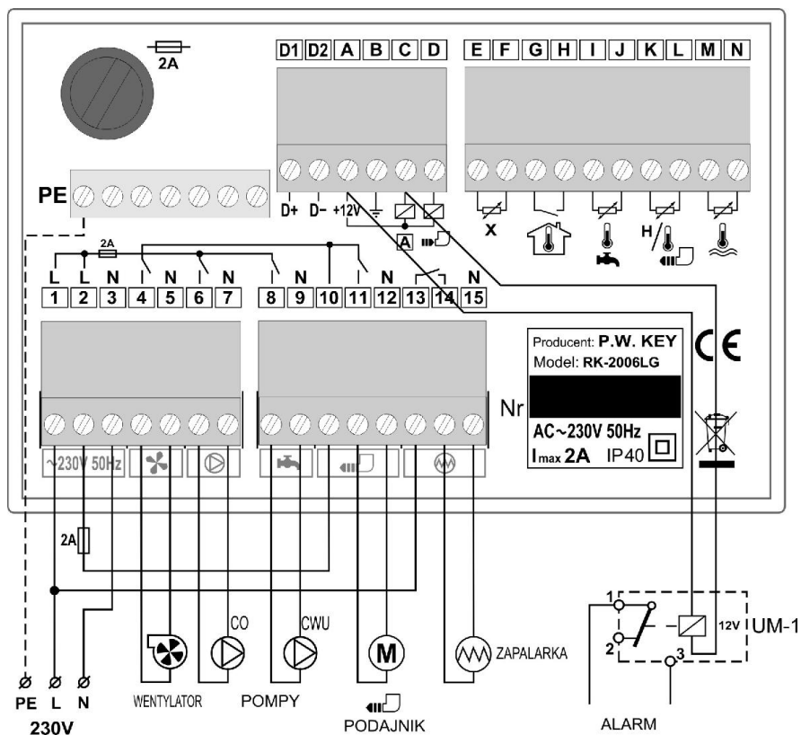
Rysunek 3. Schemat podłączenia regulatora RK-2006LG (z układem sygnalizatora alarmów).
