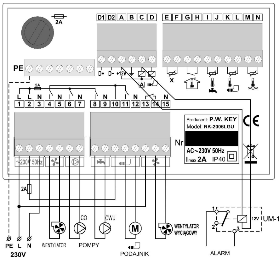
Rysunek 3. Schemat podłączenia regulatora RK-2006LGU (z układem sygnalizatora alarmów).
