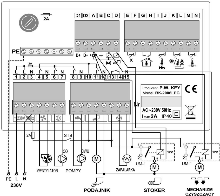
Rysunek 2. Schemat podłączenia regulatora RK-2006LPGP.
