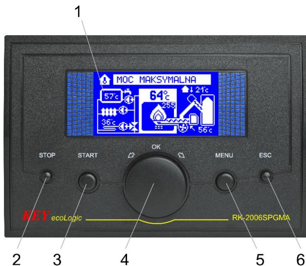
Rysunek 1. Płyta czołowa regulatora RK–2006SPGMA.
