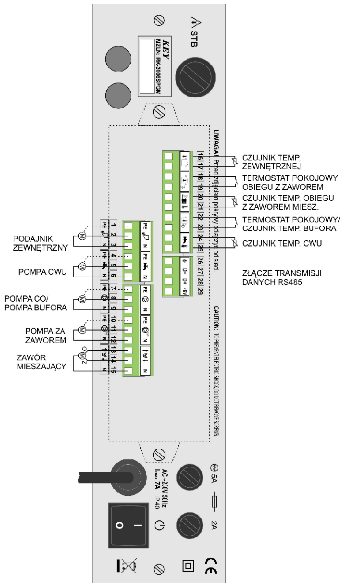
Schemat podłączenia regulatora RK-2006SPGMA z modułem zasilacza MZLN.
