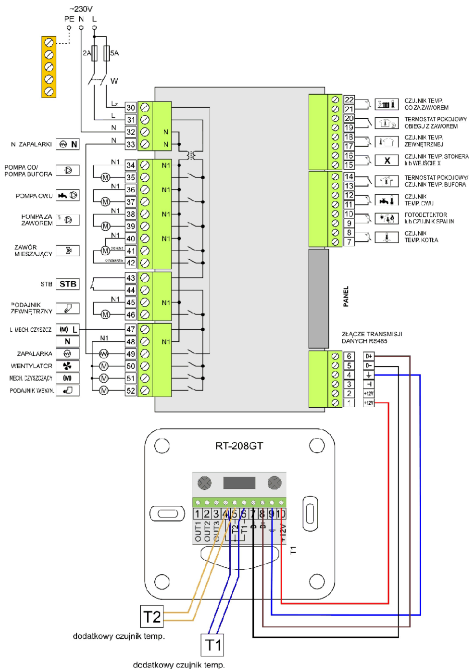
Schemat podłączenia regulatora RT-208GT do regulatora RK-2006SPGMA z modułem zasilacza MZK, MZM2.
