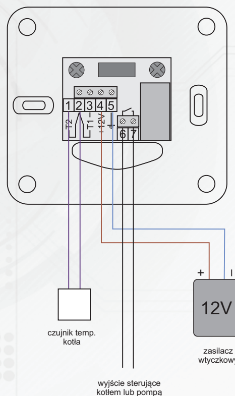
Schemat podłączenia regulatora RT-208B do regulatora kotła
